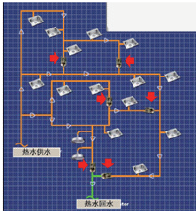
热水使用点随机分布水流示意图
