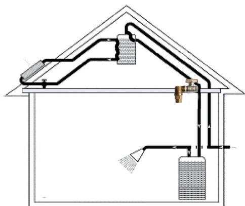
承压式平板太阳能
